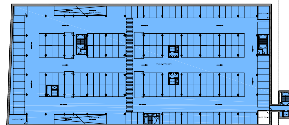
PLANTA APARCAMENT SOTERRANI -3
