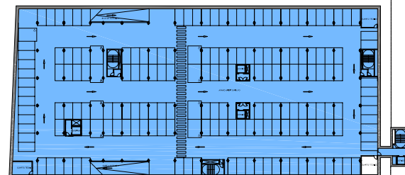
PLANTA APARCAMENT SOTERRANI -5
