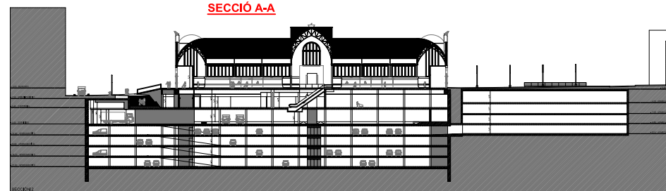
SECCIÓ A-A
